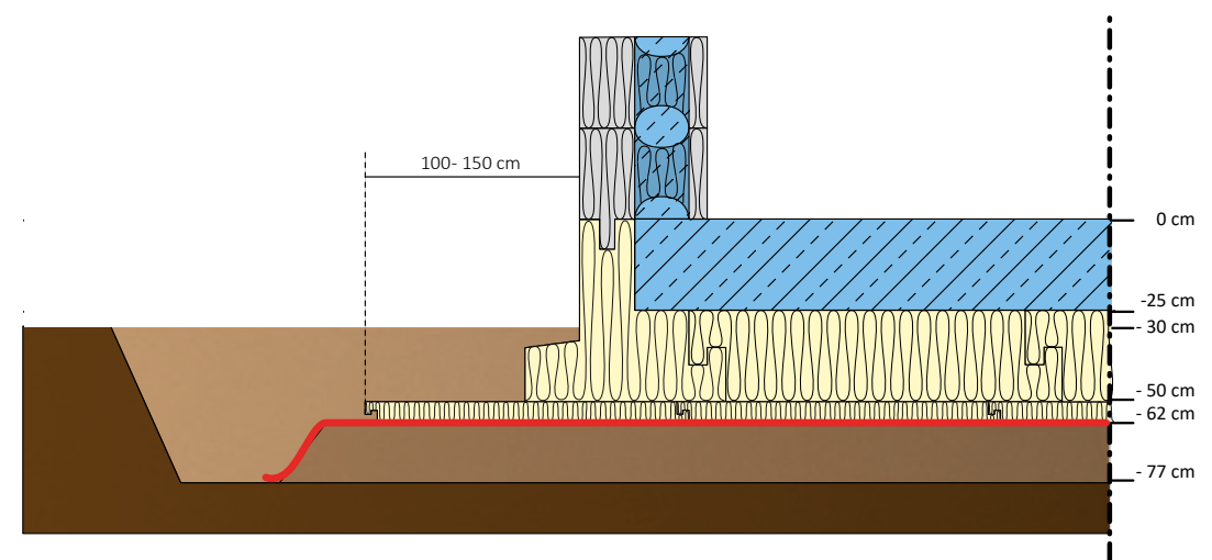
Fig. 2 Construcție schematică a fundației cu planșeu folosind izolație termică suplimentară
